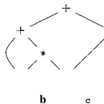
(a) DAG
