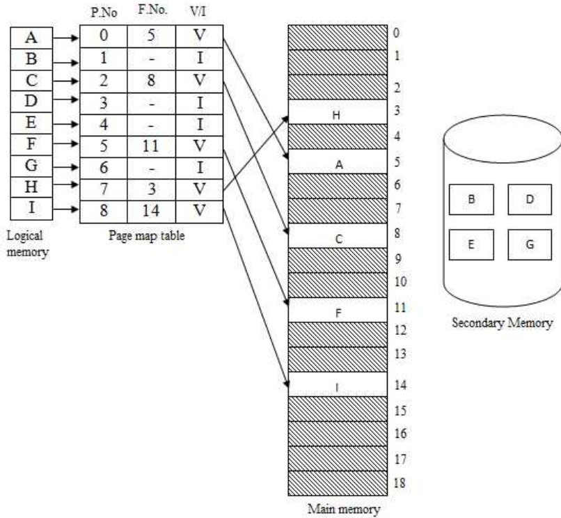
Fig.3.24: Demand Paging
